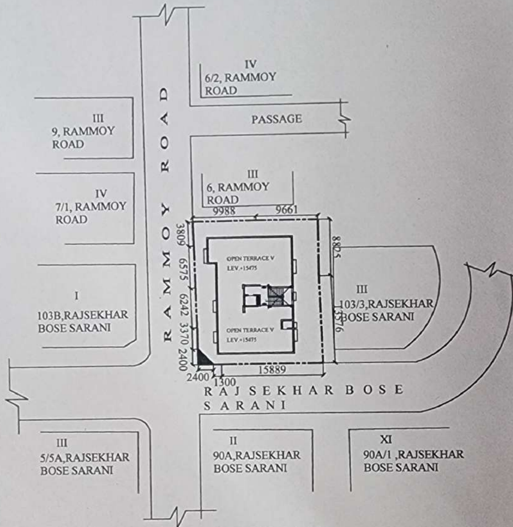
SITE PLAN SCALE-1:600
